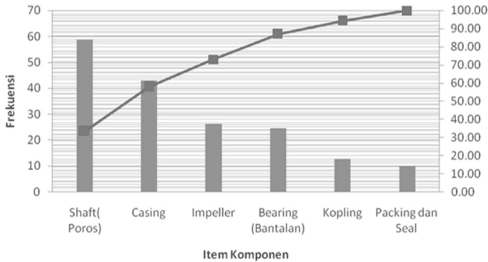
Gambar 2. Diagram Pareto Persentase Downtime Mesin Pemisah Biji Tahun Produksi Januari 2015- Desember 2015
