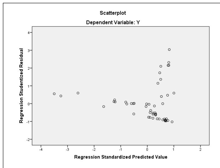
Gambar 4.3 Uji Heteroskedastisitas dengan Scatterplot
