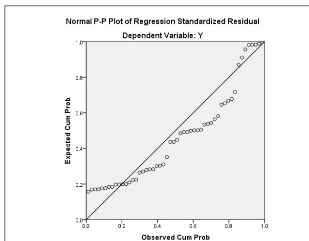
Gambar 4.2 Uji Normalitas dengan P-P Plot of Regression
